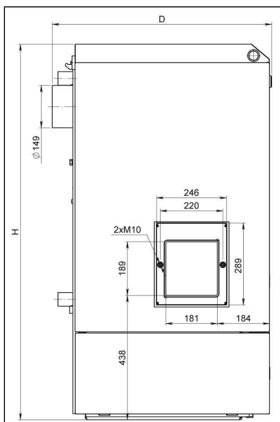
Фигура 4.2. Габаритни и присъединителни размери на водогрееен пелетен котел серия "Pelletherm V.4 LT" – поглед от към страната на фланеца за монтаж на пелетната горелка.
