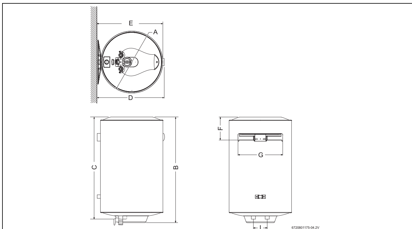
Фиг. 2 Размери в mm (ES035/050/080/100/120-4...)
