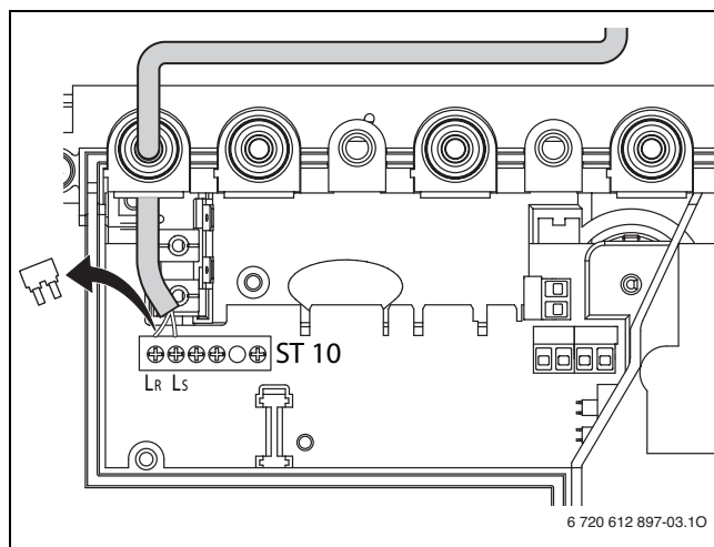
Фиг. 29 Присъединение (230 V AC, премахнете моста между L_S и L_R )
