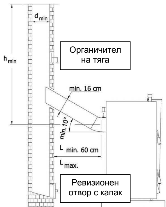
Фигура 9. Препоръчителни размери на комината система
