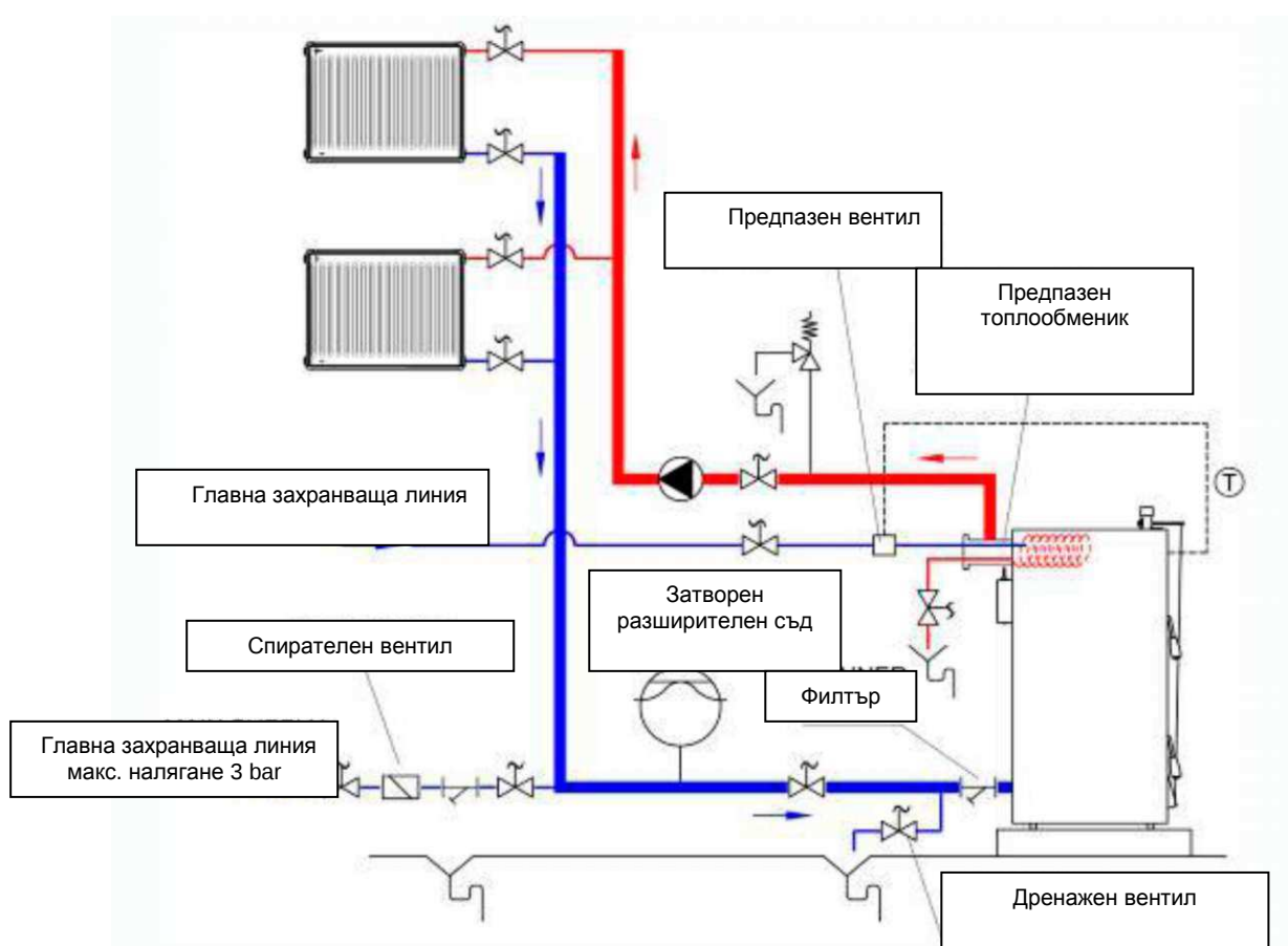
Фигура 8. Примерна принципна хидравлична схема за свързване на котел Bisolid N към отоплителна система със затворен разширителен съд
