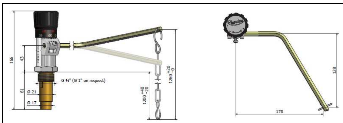
Фигура 4. Монтажни и габаритни размери на терморегулатора на мощността
