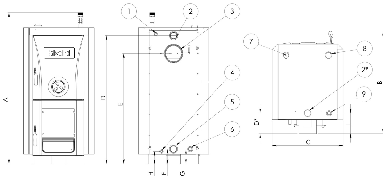
Фигура 1. Габаритни и присъединителни рамери на котел Bisolid N
