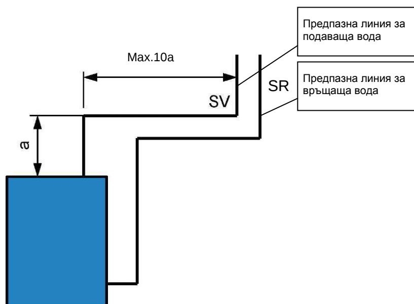
Фигура 7. Изисквания към разширителния съд
