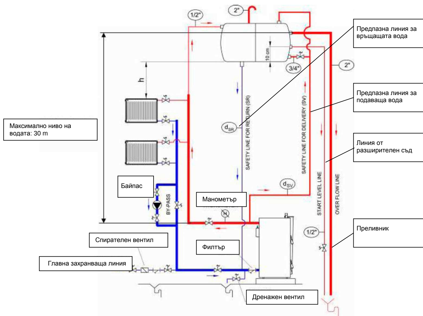
Фигура 6. Препоръчана хидравлична схема с отворен разширителен съд
